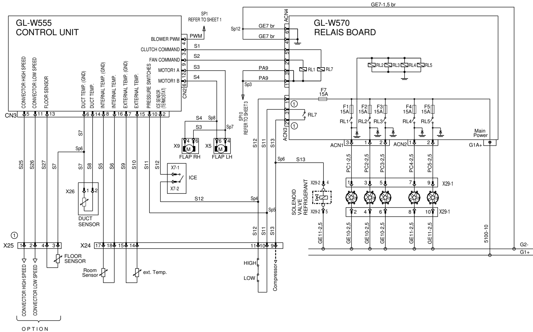
Abb. 10 Wiring Diagram / Schéma zapojení (Page 2 of 6)
